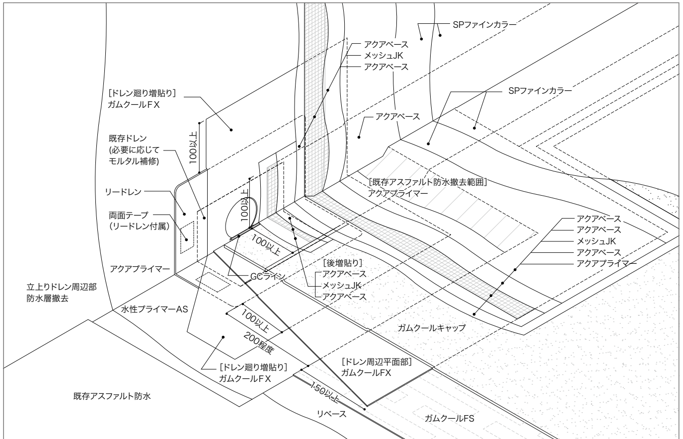
改修用ドレン(横)塗膜防水併用工法GSS-2S/立上りAQ-160(アクアベース後増貼り)
