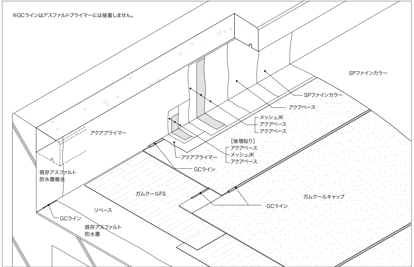
立上り塗膜防水併用工法GSS-2S/立上りAQ-160(アクアベース後増貼り)
