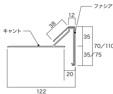
フラッシュエッジ110A (単位:mm)
