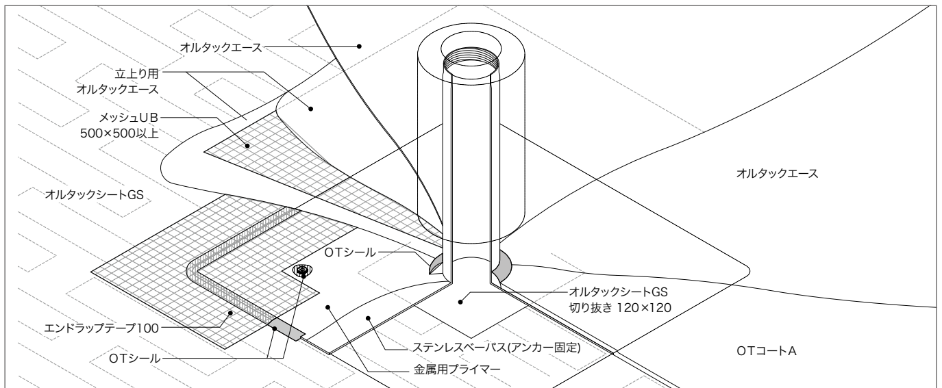
脱気筒：ステンレスペーパス
