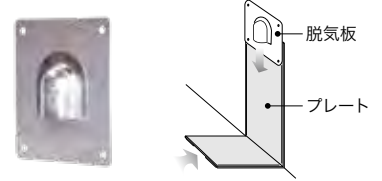
立上り用ステンレスペーパス
