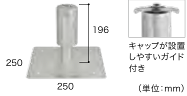
ステンレスペーパスⅡ
