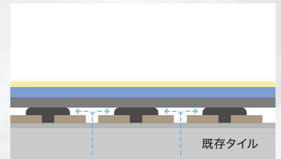
パネルの点接着固定により下地水分を拡散
