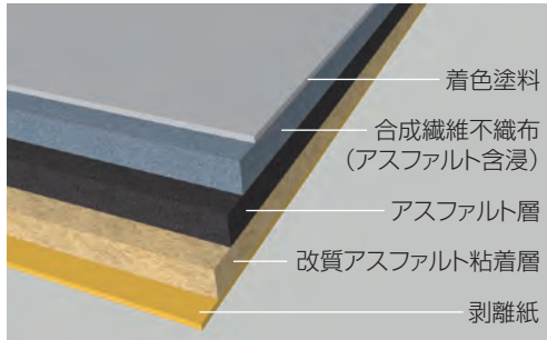
【構成図】
