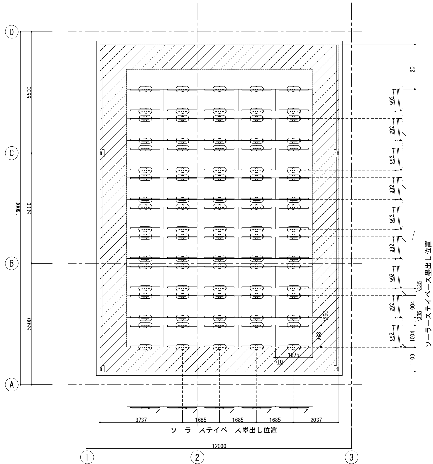
屋根伏図
